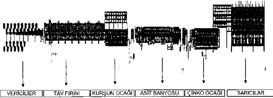
Resim 11/12: Rozet Galvanizli Tel
